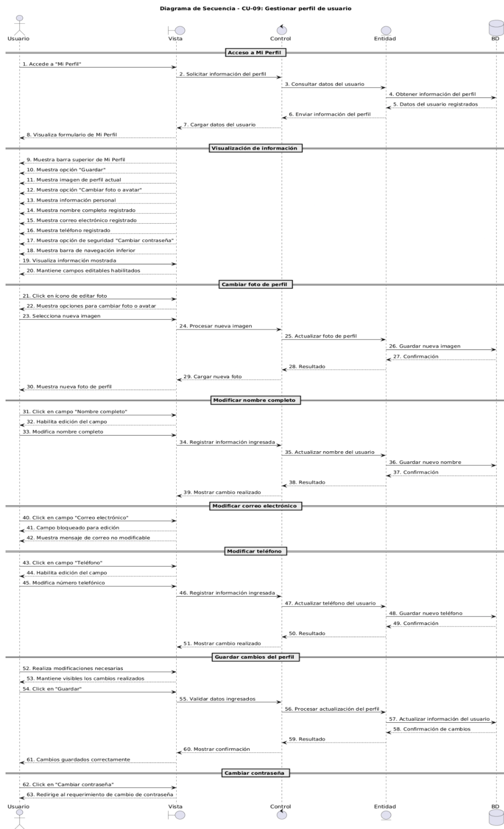
Figura 30. Diagrama de Secuencia CU-09 “Gestionar perfil de usuario”
