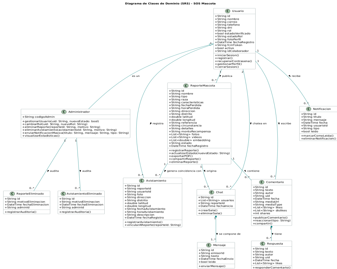
Figura 39. Diagrama de Clases del Sistema SOS Mascota
