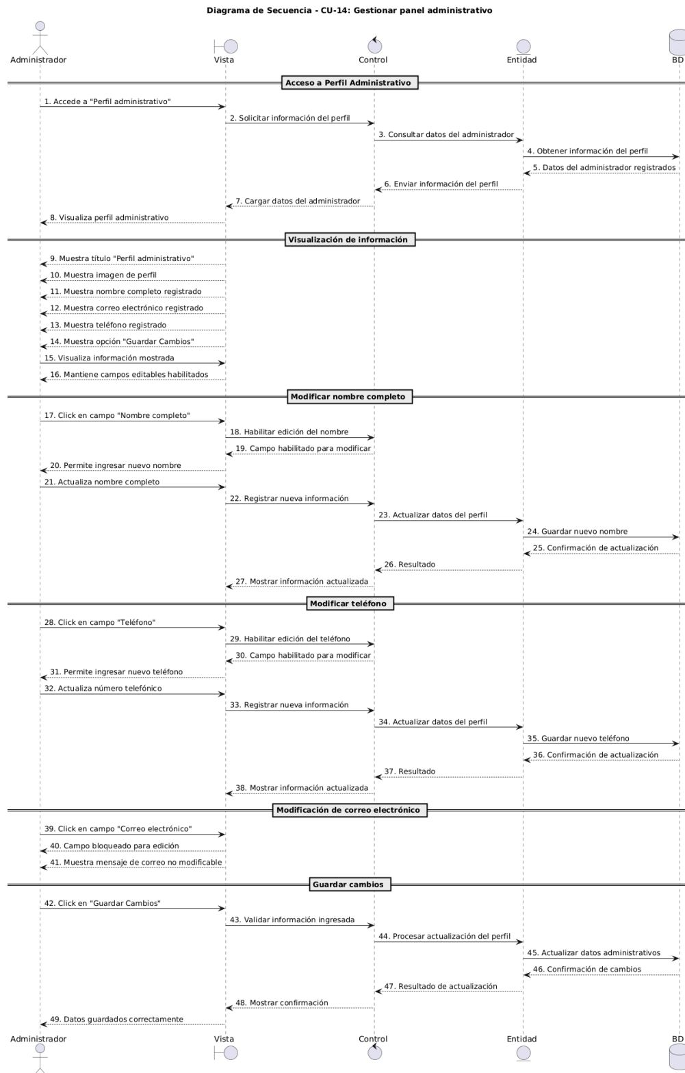
Figura 35. Diagrama de Secuencia CU-14 “Gestionar panel administrativo”
