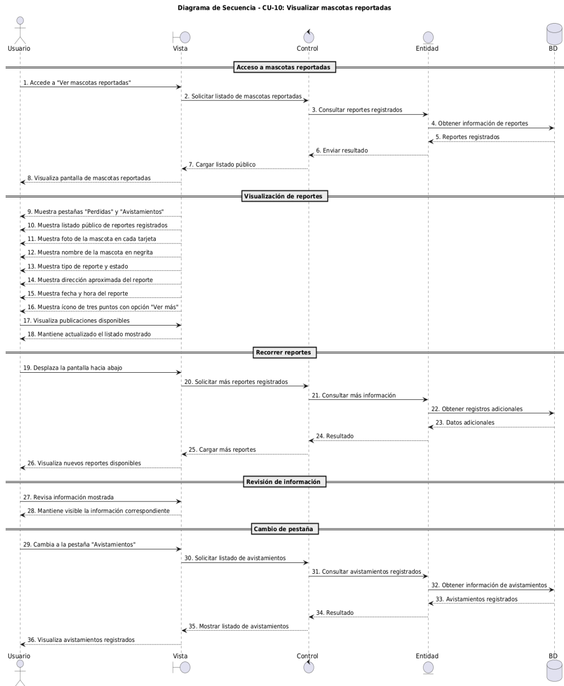
Figura 31. Diagrama de Secuencia CU-10 “Visualizar mascotas reportadas”
