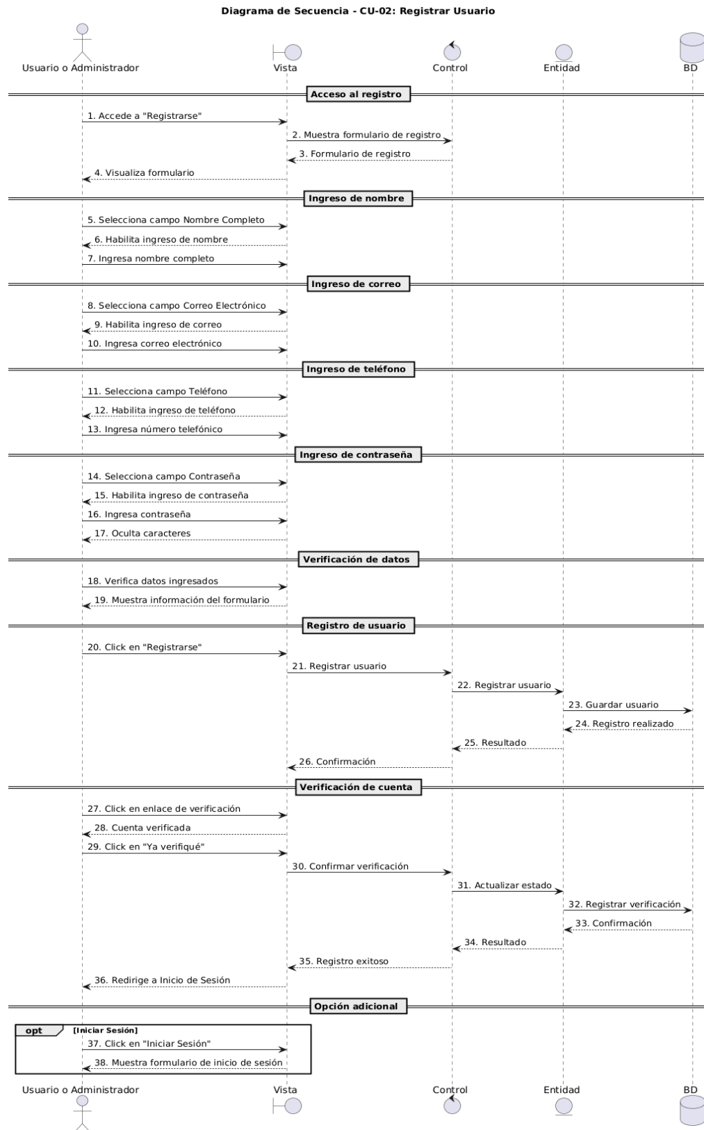
Figura 23. Diagrama de Secuencia CU-02 “Registrar usuario”
