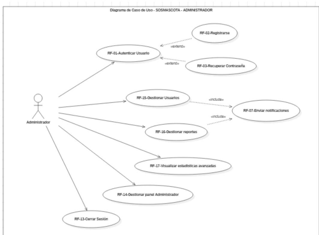
Figura 07. Diagrama de Casos de Uso-Administrador-SOSMascota
