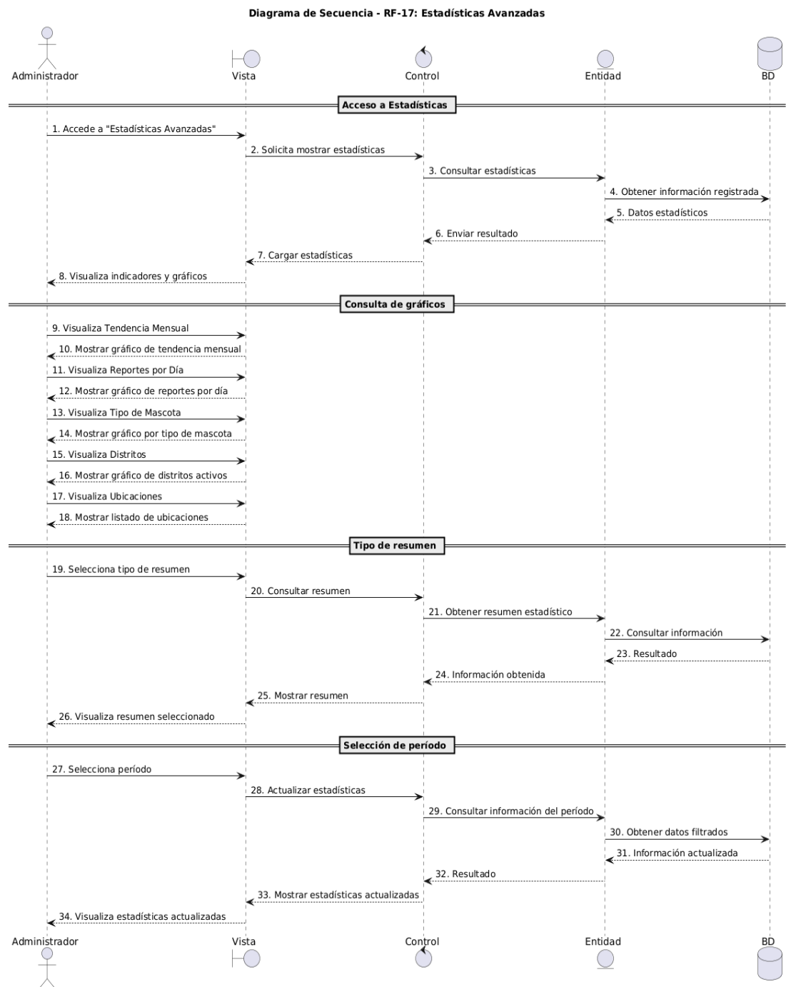
Figura 38. Diagrama de Secuencia CU-17 “Visualizar estadísticas avanzadas”
