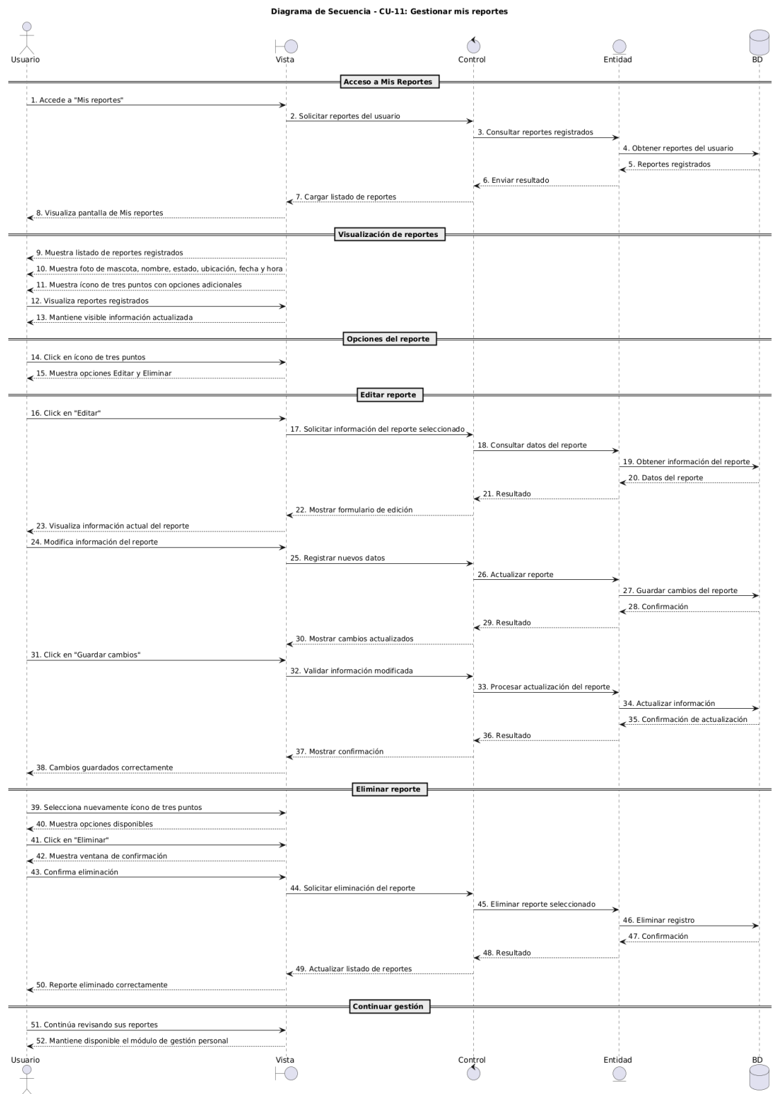
Figura 32. Diagrama de Secuencia CU-11 “Gestionar mis reportes”
