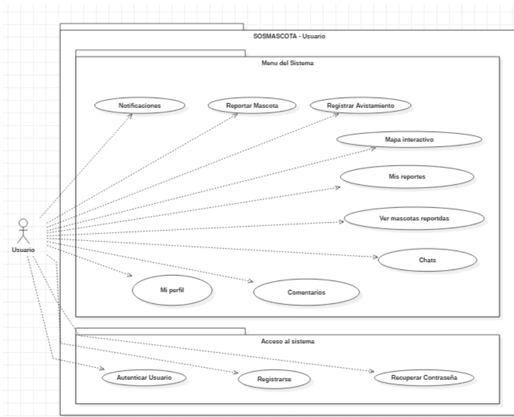
Figura 04. Diagrama de Paquete de la aplicación móvil SOS Mascota - Usuario
