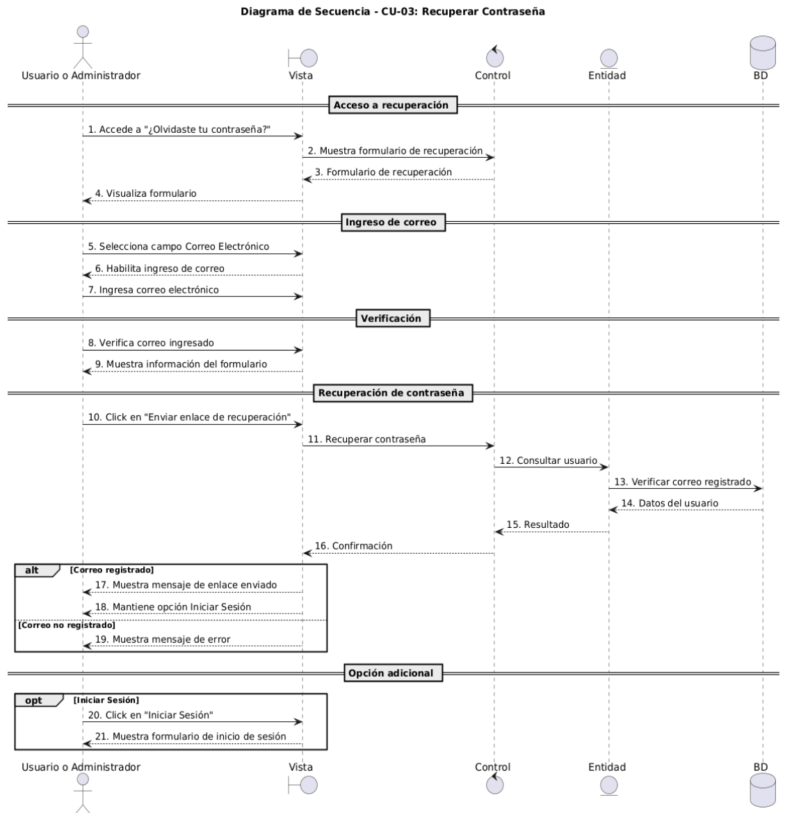
Figura 24. Diagrama de Secuencia CU-03 “Recuperar Contraseña”
