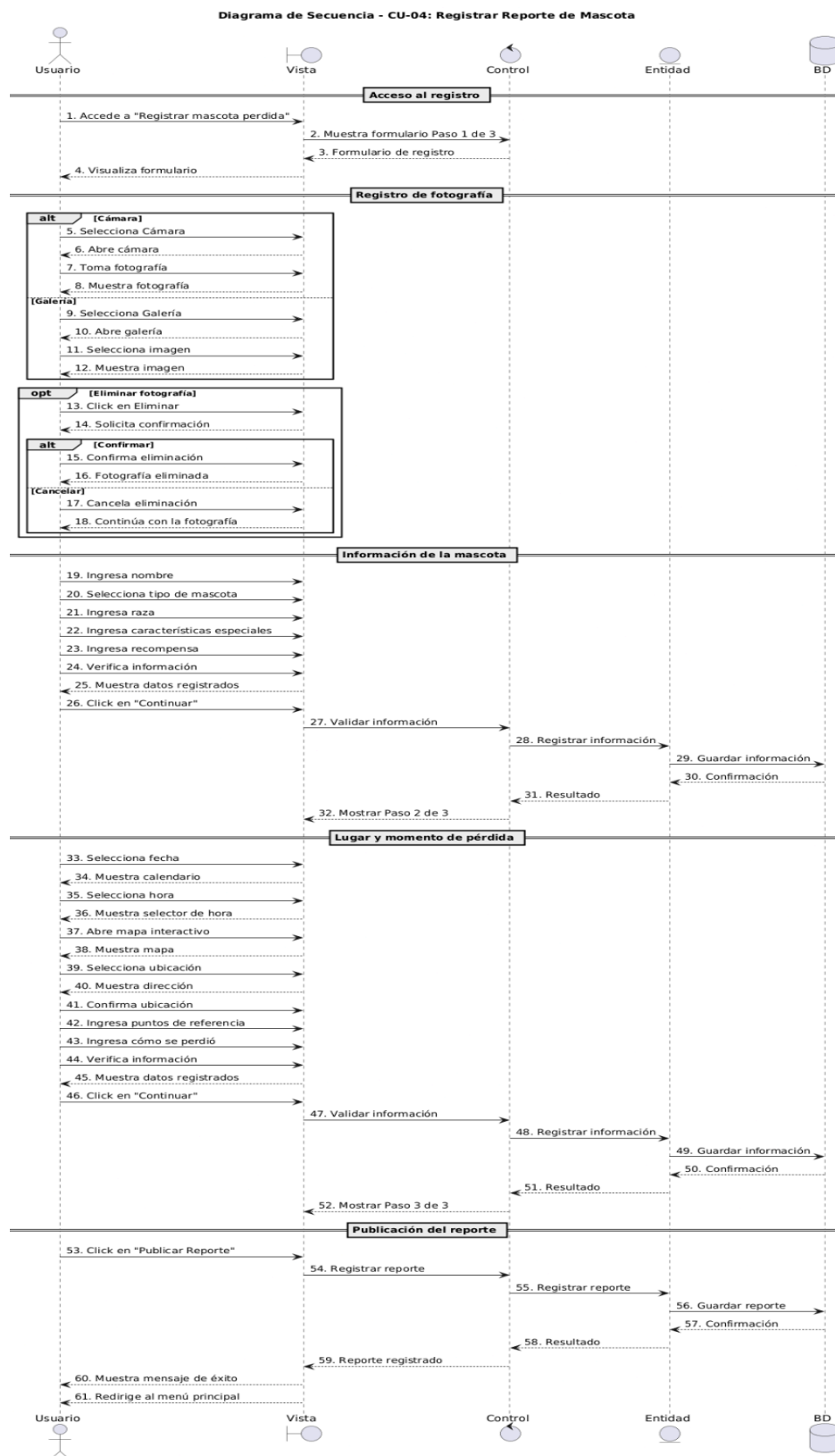
Figura 25. Diagrama de Secuencia CU-04 “Registrar reporte de mascota”
