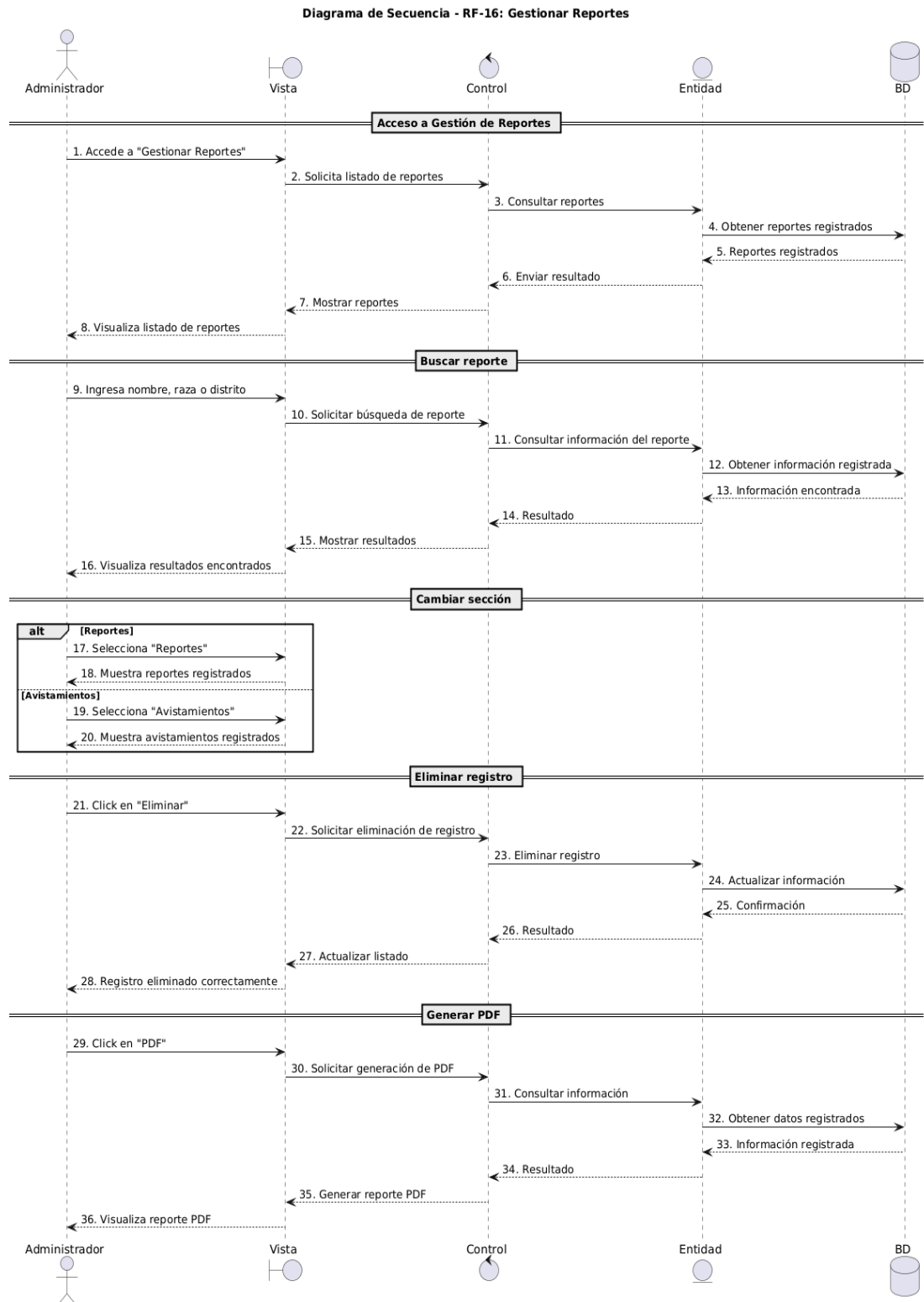
Figura 37. Diagrama de Secuencia CU-16 “Gestionar reportes”
