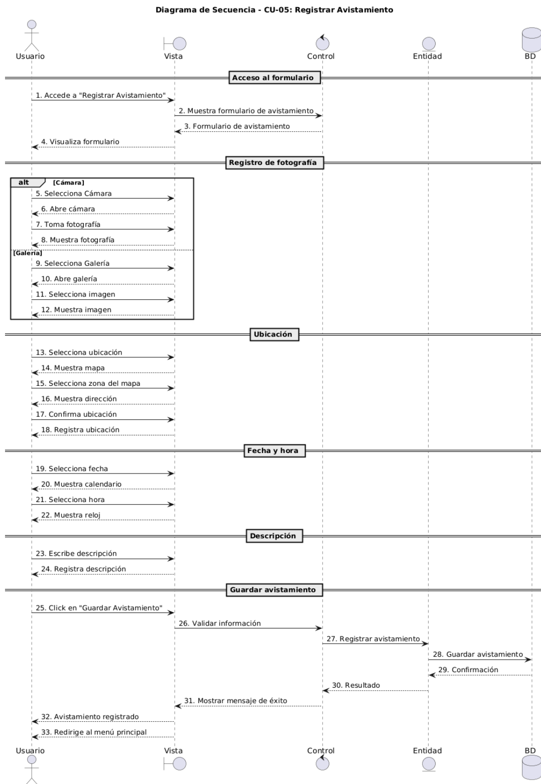
Figura 26. Diagrama de Secuencia CU-05 “Registrar avistamiento de mascota”
